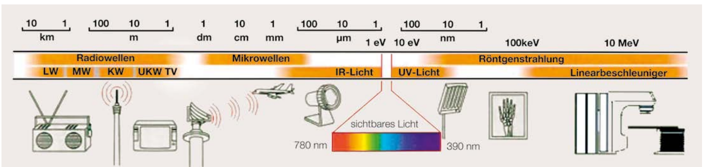
Abb. 4: Die Photonenstrahlung gehört zu den elektromagnetischen Wellen ebenso wie Radiowellen, Mikrowellen, Licht und Röntgenstrahlung. Die Durchdringungskraft dieser Strahlung ist aber größer und auch die deponierte Energie pro Absorptionsprozess ist weit höher, als bei den anderen aufgezählten elektromagnetischen Wellen. (Prolight GmbH1, 11)
